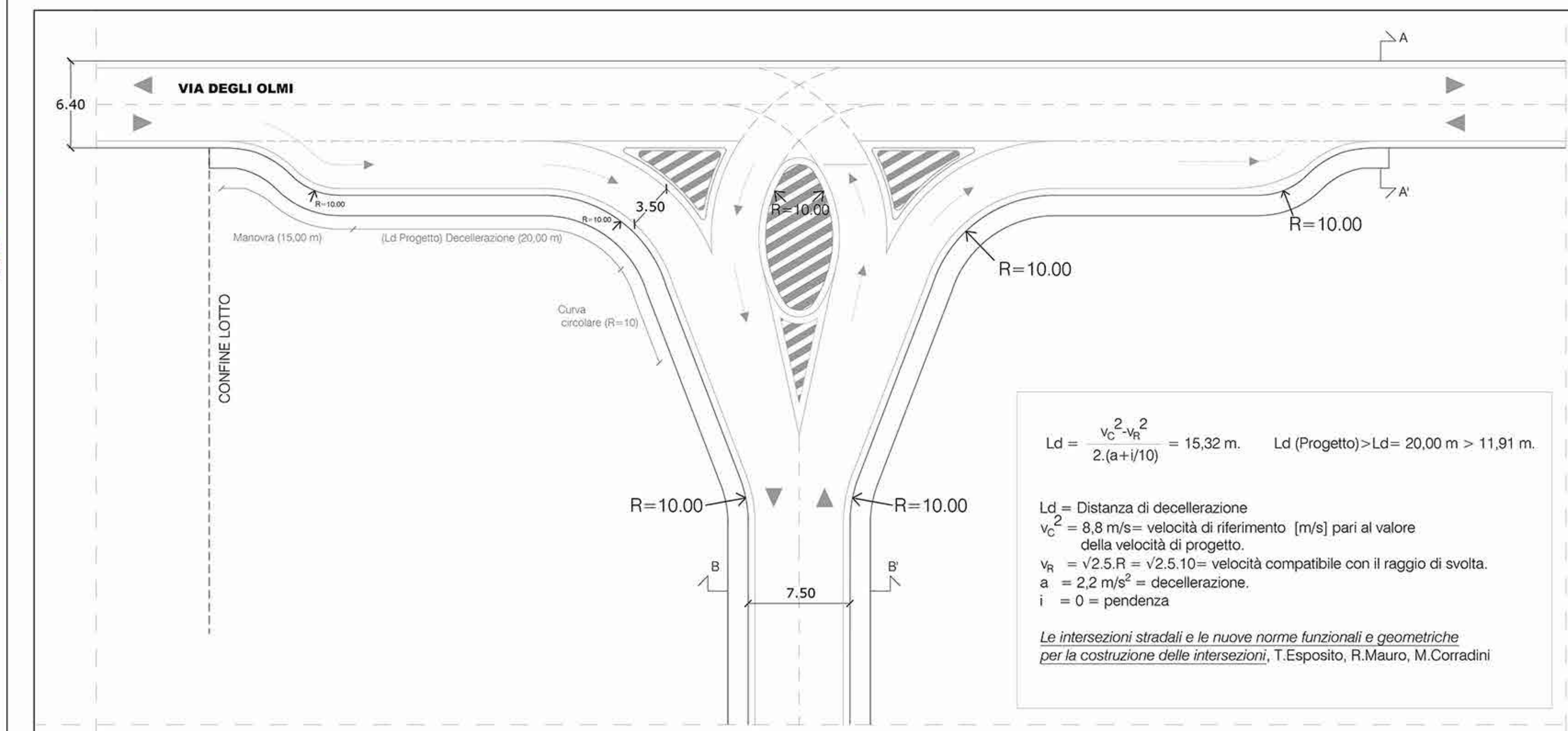
NUOVO INCROCIO VIA DEGLI OLMI - SCALA 1:200
