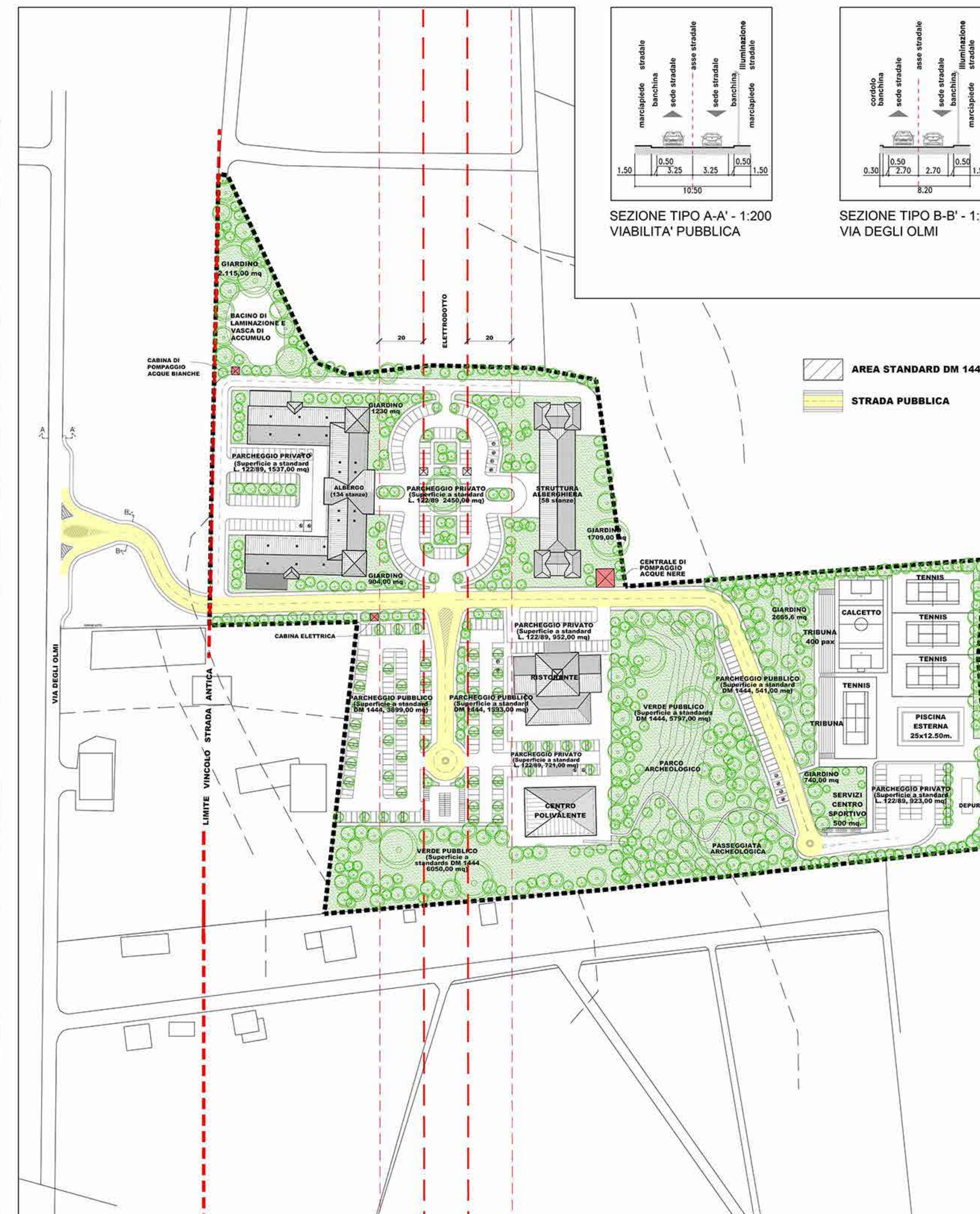
PLANIMETRIA DI INTERVENTO - SCALA 1:1.00
